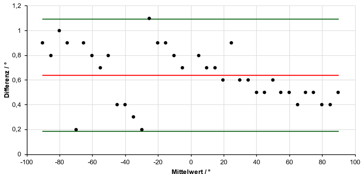
Abbildung 5: Vergleich der Winkelmessung mit dem Zebris-System und den DOTs für die Ulnar- und Radialabduktion. Die rote Linie visualisiert den Mittelwert der Differenzen, die grünen Linien stellen die Übereinstimmungsgrenzen dar.
