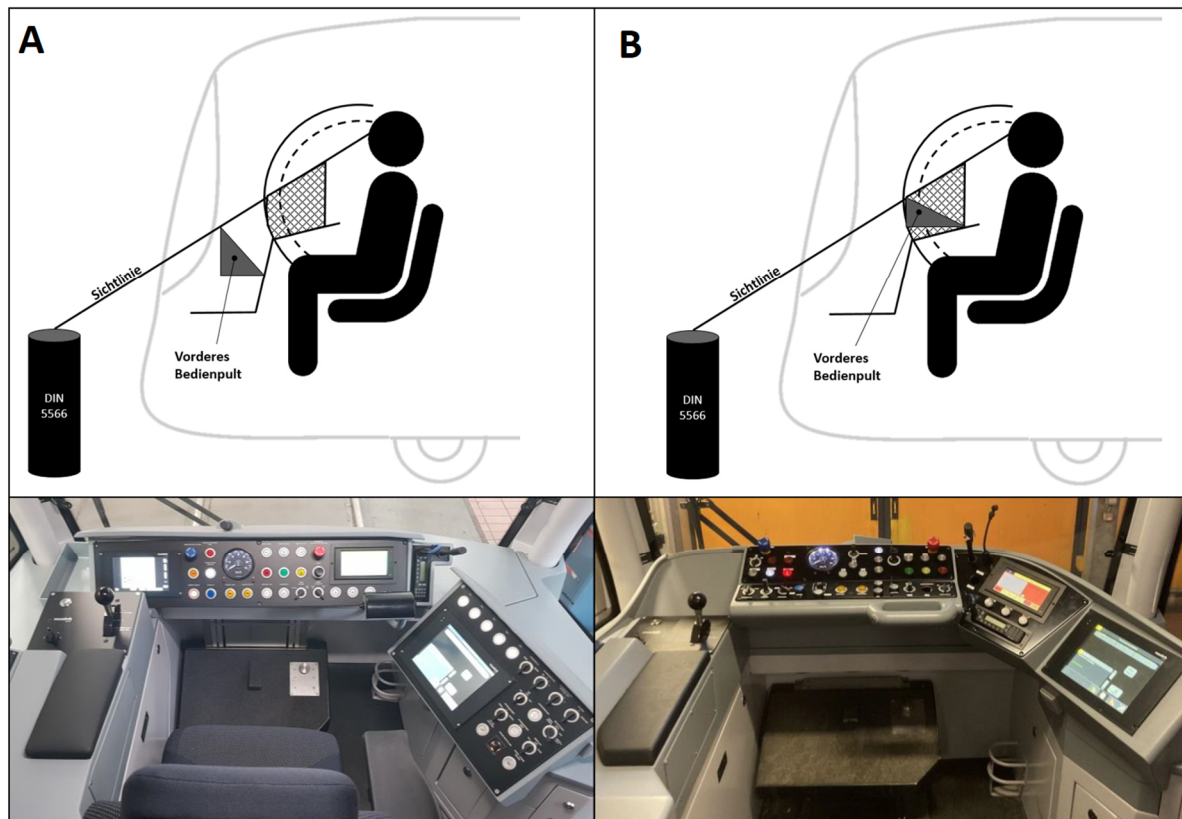
Abbildung 2: (A) Schematische Darstellung der Positionierung des vorderen Bedienpults im NET2012 (oben) und Draufsicht auf den NET2012-Führerstand (unten), (B) Schematische Darstellung der Positionierung des vorderen Bedienpults im neuen Prototyp (oben) und Draufsicht auf den neuen Führerstand (unten).
