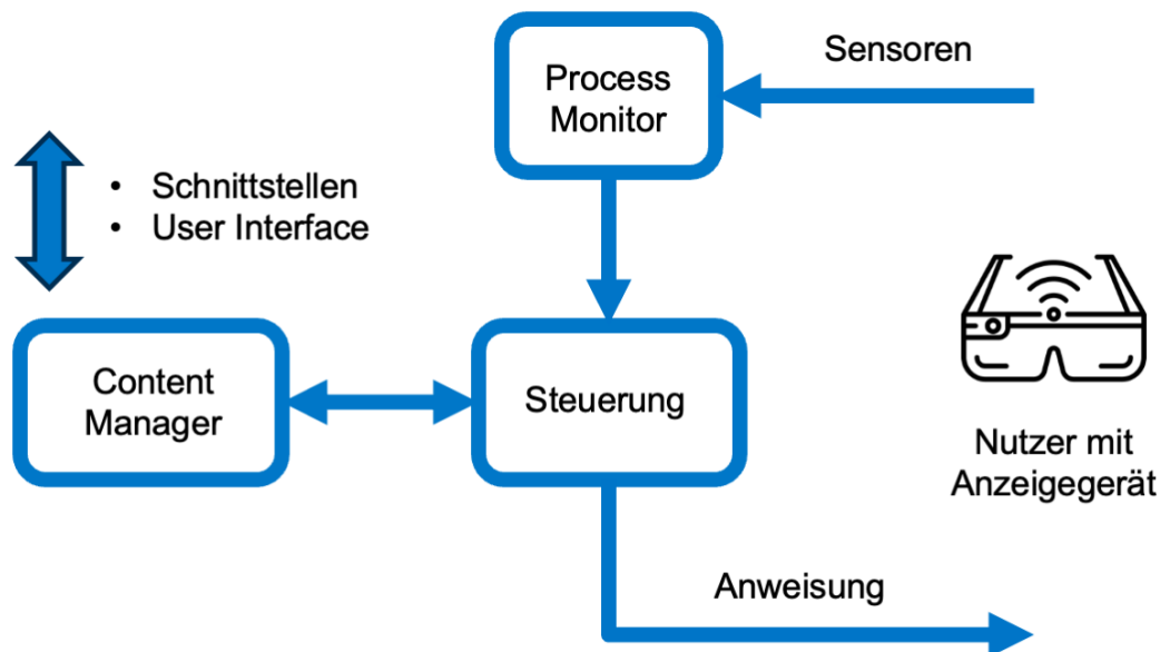
Abbildung 1: Schematische Darstellung kontextsensitiver Assistenzsysteme mit den Hauptkomponenten als Kästchen dargestellt.
