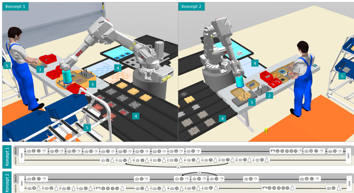
Abbildung 4: Aufbau MRI-Arbeitsplätze (1: Vormontage, 2: Vormontage BG Druck- Feder- & Endplatte, 3: Drehtisch, 4: Zuführsysteme für Roboter 5: manuelle Zuführung (IST) inkl. Arbeitsgangfolge-Diagramme für MRI-Konzept 1 und MRI-Konzept 2
