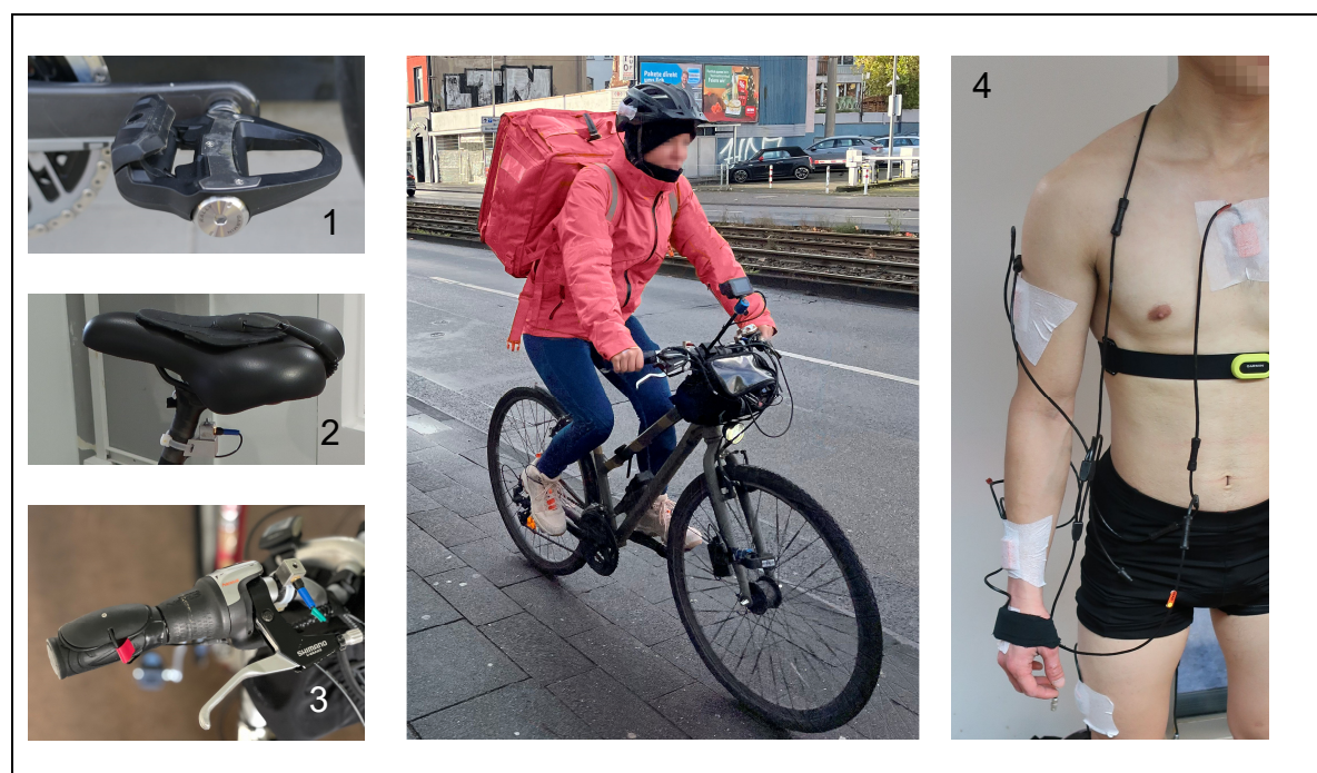
Abbildung 1: Untersuchung der mechanischen und physikalischen Expositionen; 1: Garmin Rally RS200 Powermeter, 2: Beschleunigungsaufnehmer auf dem Sattel und Sattelstütze, 3: beschleunigungsaufnehmer auf dem Lenkergriff und Lenkerstange, 4: Anbringung der IMU- Sensoren am Körper.
