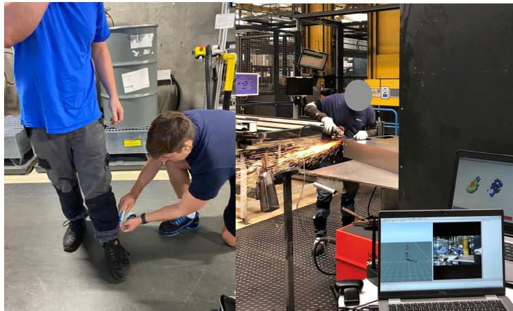
Abbildung 2: Kinematische und kinetische Analyse von Produktionsarbeitern mit inertialer Messensorik und plantarer Innenschuh-Messung.
