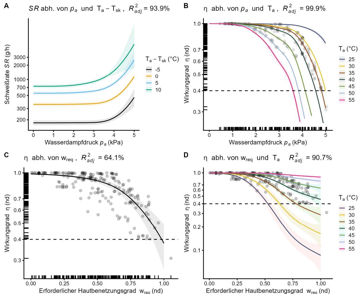
Abbildung 4: (A) Mittels an den gesamten Datensatz angepasster monotoner Spline-Funktionen durch Wasserdampfdruck ( p_a ) und den Gradienten zwischen Luft- und Hauttemperatur ( T_a - T_{sk} ) vorhergesagte, logarithmisch skalierte Schweißraten (SR) mit 95 %-Konfidenzband und nach der Parameteranzahl adjustiertem R^2_{adj} als Maß der Anpassungsgüte; sowie der daraus bestimmte Wirkungsgrad der Schweißverdunstung ( \eta ) abhängig von (B) p_a und T_a ; (C) erforderlichem Hautbenetzungsgrad ( w_{\text{req}} ); (D) w_{\text{req}} und T_a .
