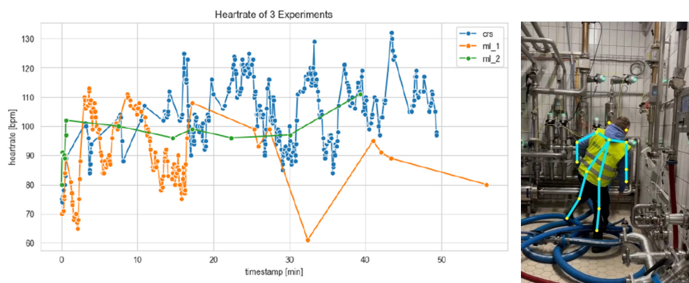
Abbildung 2: Darstellung der Herzfrequenz aus drei Messreihen an der bestehenden Mischanlage, sowie die Auswertung aus dem videobasierten Ansatz
