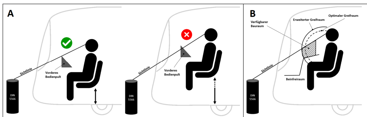
Abbildung 1: (A) Schematische Darstellung der veränderten Sichtbedingung bei erhöhter Sitzposition, (B) Schematische Darstellung des Bauraums bedingt durch ergonomische Vorgaben gemäß DIN 5566.
