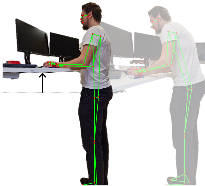
Abbildung 1: Visualisierung des Artefakts. Wenn die Arbeitspose als unergonomisch evaluiert wird, passt sich die Tischhöhe an, bis die Körperhaltung durch die Anpassung adaptiert wird.
