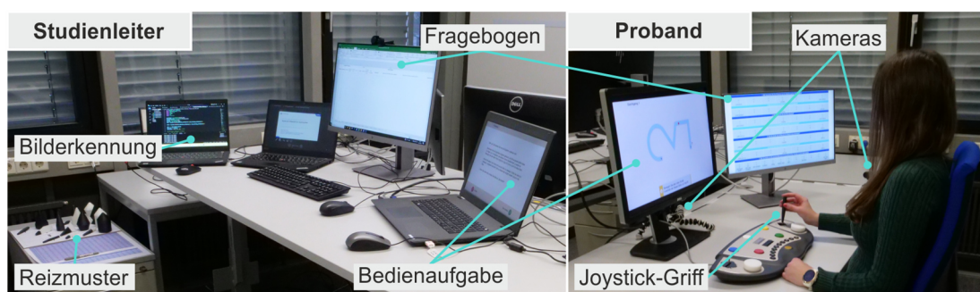
Abbildung 2: Versuchsaufbau für Studienleiter (links) und Probanden (rechts).
