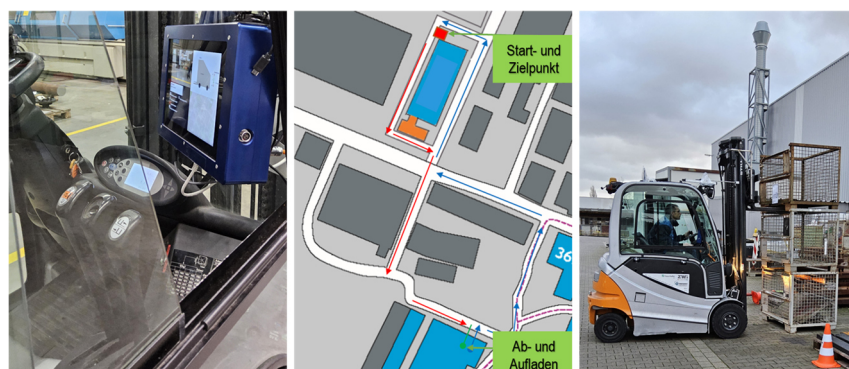
Abbildung 1: Praxistest: Stapler mit App (links), Testparcours (Mitte) und Testfahrt (rechts).
