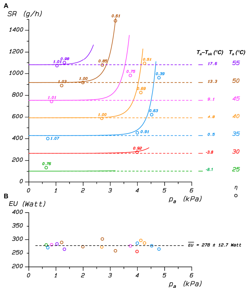
Abbildung 2: (A) Schweißrate (SR) in Abhängigkeit vom Wasserdampfdruck ( p_a ) längs einer Linie ( T_a - T_{sk} ) = const., die für eine vorgegebene Lufttemperatur ( T_a ) bei p_a=0 beginnt (vgl. Abb. 1D) mit abgeleitetem Wirkungsgrad ( \eta ) für die jeweiligen Messpunkte bei T_a , und (B) Energieumsatz (EU) abhängig von p_a mit Mittelwert ( \overline{EU} ) \pm Standardabweichung für die Daten aus Abb. 1.
