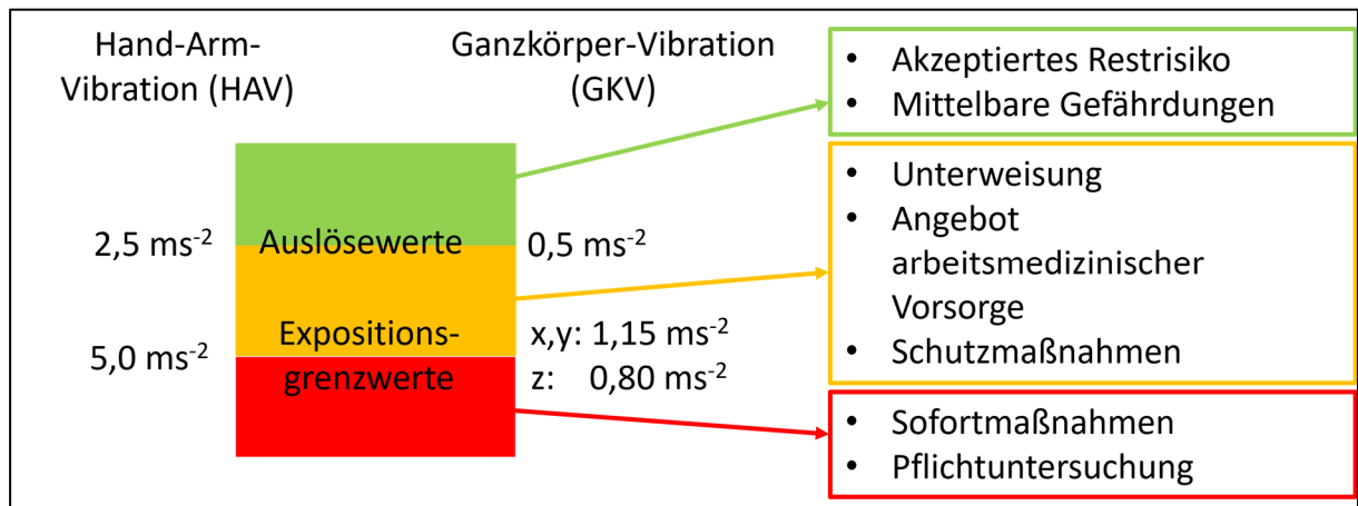
Abbildung 2: Auslöse- und Grenzwerte für eine Tages-Vibrationsexposition nach Vibrations-Arbeitsschutzverordnung für Ganzkörper- und Hand-Arm-Vibrationen mit dazugehörigen erforderlichen Präventionsmaßnahmen.
