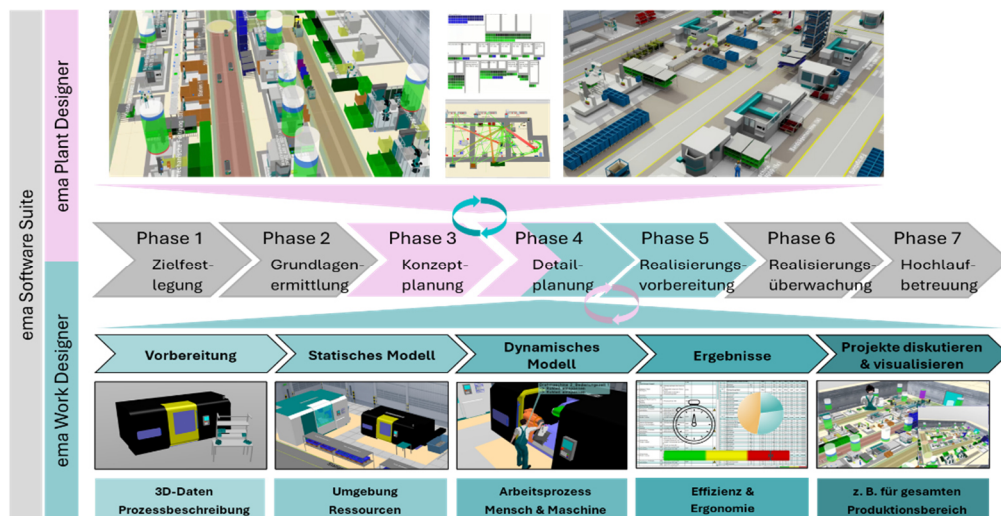
Abbildung 1: Vorgehensweise zur Planung der Fertigung von Gepäckablagefächern mittels emaSWS.
