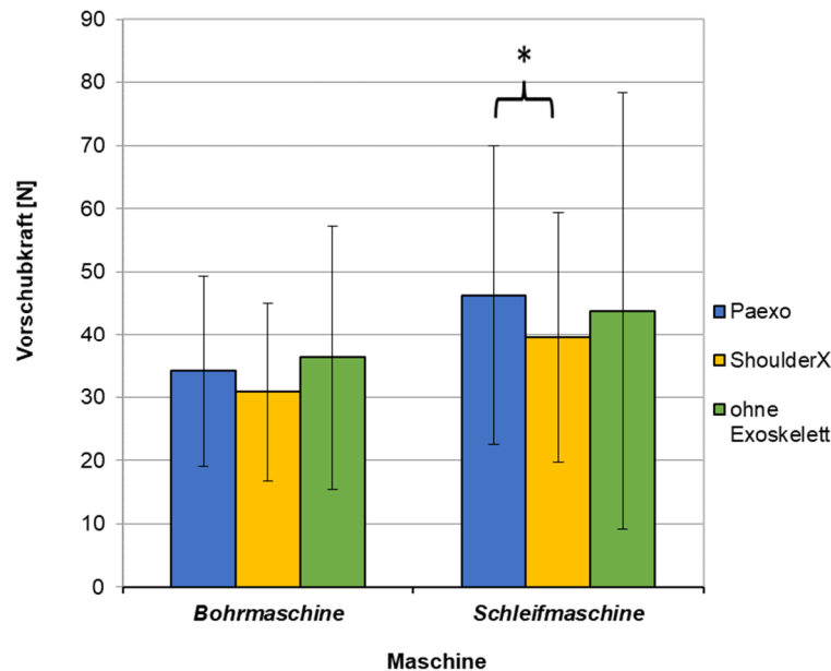
Abbildung 2: Resultierende Vorschubkraft der Maschinen mit dem Werkstück mit und ohne Exoskelette.
