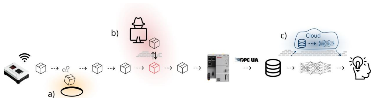
Abbildung 2: Informationsverarbeitung vom Sensor bis zum Analysemodell mit drei cybersicherheitsrelevanten Bereichen: a) Integrität der Datenerfassung, b) Verfügbarkeit und Manipulation von Daten, c) Datenhoheit in der Cloud
