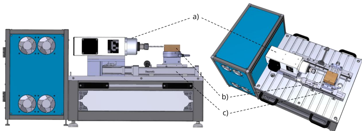
Abbildung 1: Mobiler Demonstrator LOTTA des LWM der TU Dresden. a) Spindel, b) Werkstück, c) Vorschubachse.
