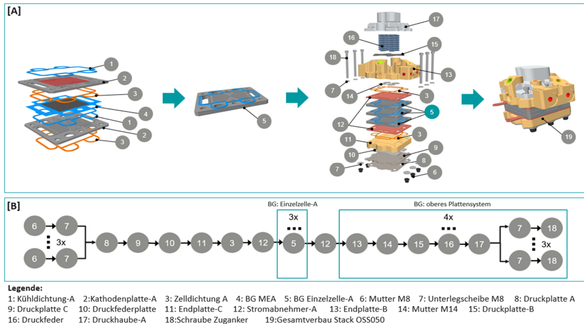
Abbildung 2: Zusammenbau OSS050-Stack mit Einzelkomponenten und BZ-Einzelzelle [A] sowie Montagevorranggraphen [B]
