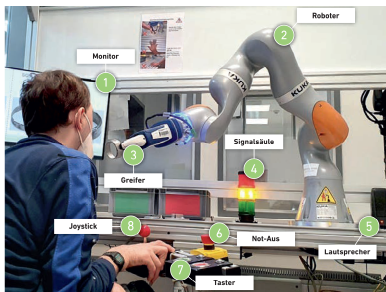
Abbildung 2: Arbeitsplatz mit kollaborativer Anwendung zur optischen Qualitätsprüfung aus dem NextGeneration Projekt. (Niedziella et al. 2022).
