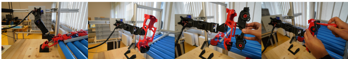
Abbildung 2: Unterstützende Tätigkeit des MRK-Systems während der Montage.
