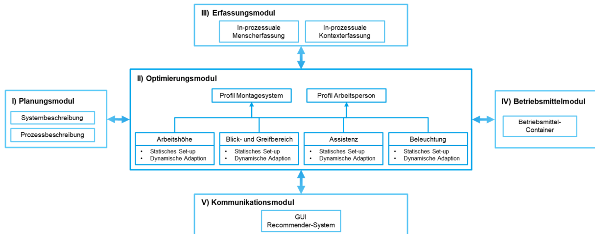
Abbildung 1: Grundlegender Aufbau des Software-Frameworks des Recommender-Systems.
