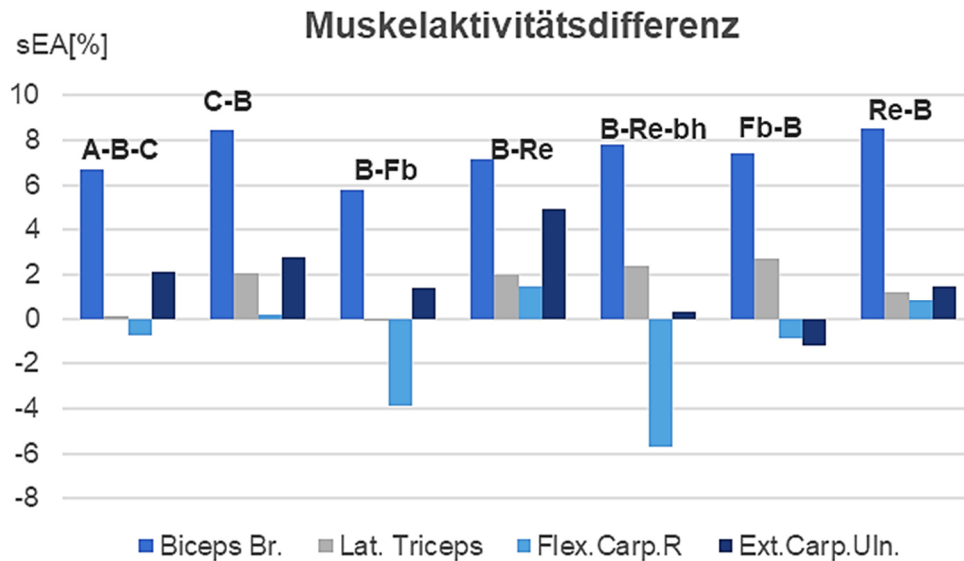
Abbildung 3: Muskelaktivitätsdifferenzen des rechten Hand-Arm-Systems beim Umsetzen der Kiste. Die Ermittlung zeigt die Differenz zwischen VP01 und VP02.
