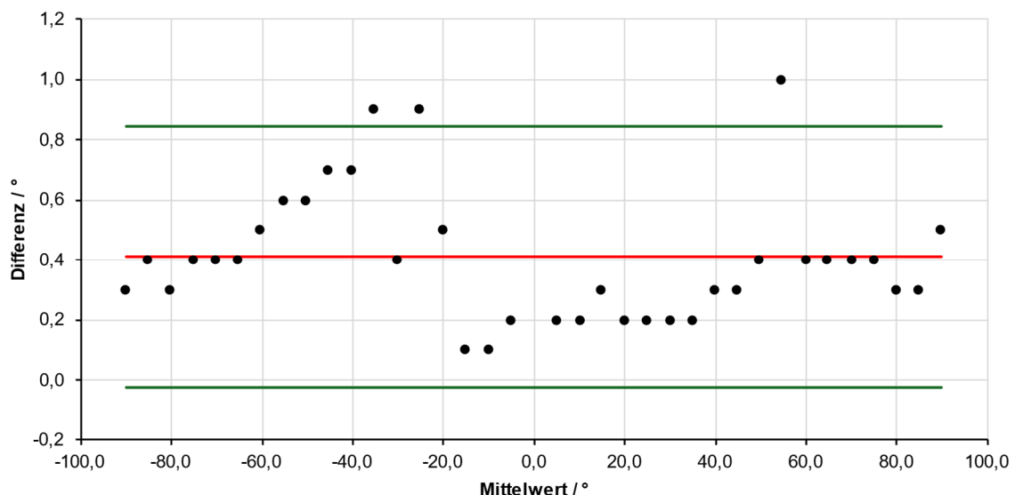
Abbildung 4: Vergleich der Winkelmessung mit dem Zebri-System und den DOTs für die Palmarflexion und Dorsalextension. Die rote Linie visualisiert den Mittelwert der Differenzen, die grünen Linien stellen die Übereinstimmungsgrenzen dar.
