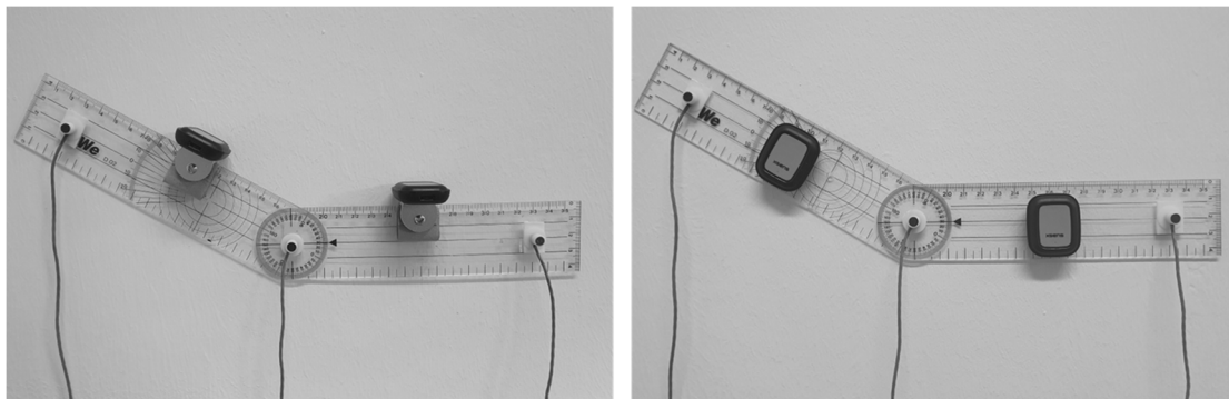
Abbildung 1: Testaufbau für die Validierung: Platzierung der DOTs sowie der Marker auf dem Goniometer für (links) die Dorsalextension und Palmarflexion (hier 30^\circ Dorsalextension); (rechts) Ulnar- und Radialabduktion (hier 30^\circ Ulnarabduktion).
