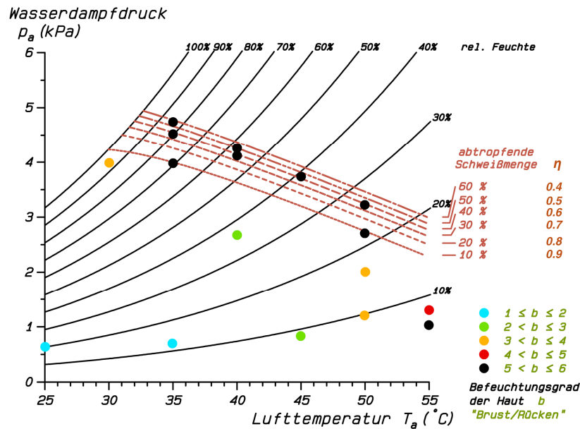
Abbildung 3: Psychrometrisches Diagramm mit Linien gleicher Abtropfraten bzw. Wirkungsgrades ( \eta ) des Schweißes und Einstufung des Hautzustandes (1: „Fühlt sich trocken an, sieht matt aus“; 2: „Fühlt sich feucht an, sieht nicht glänzend aus“; 3: „Glänzend, noch keine deutlichen Schweißtropfen“; 4: „Deutlich sichtbare Schweißtropfen“; 5: „Herablaufende Schweißtropfen“; 6: „Abtropfen von Schweiß“) an allen Messpunkten eines Probanden. Der Mittelwert der Einstufungen von Brust und Rücken wurde für die Darstellung gewählt, weil Arme und Beine sich beim Gehen schneller bewegen als die Luftgeschwindigkeit und daher geringere Abtropfraten haben.
