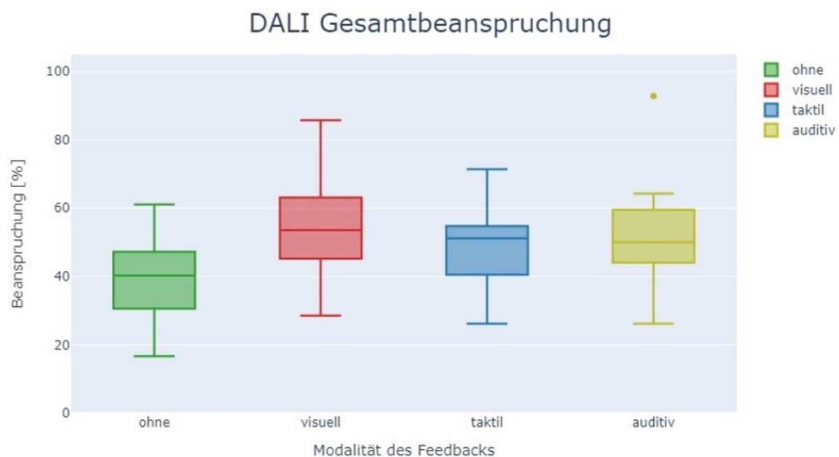
Abbildung 4: DALI Gesamtbeanspruchung.
