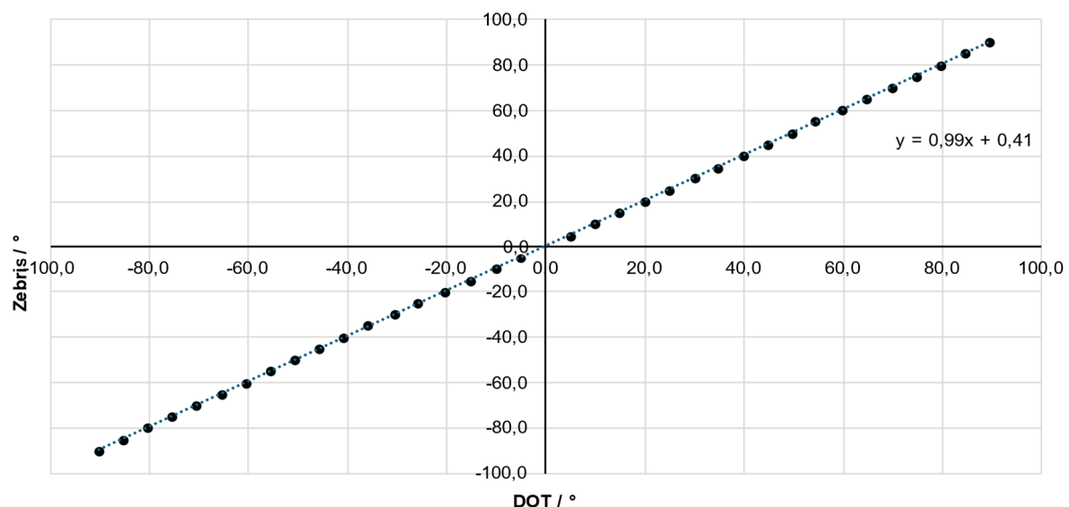
Abbildung 2: Zusammenhang zwischen der Winkelmessung mit den DOTs und dem Zebris System für die Palmarflexion (negative Werte) und Dorsalextension (positive Werte) mit linearer Regressionsgrade.
