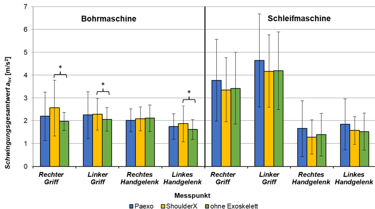
Abbildung 1: Schwingungsgesamtwert a_{hv} an den Maschinengriffen und am Handgelenk mit und ohne Exoskelette
